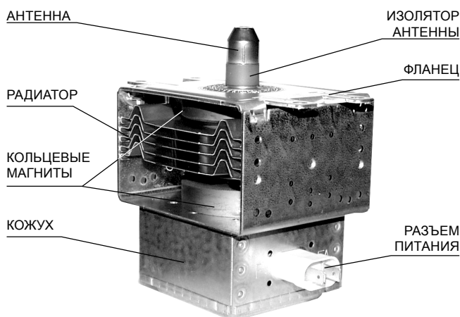
Рис. 3. Внешний вид магнетрона
